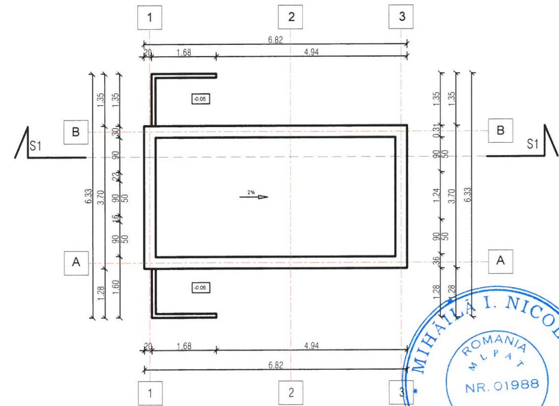
Wc public Daia - Plan învelitoare Public WC Daia - Roof floor
