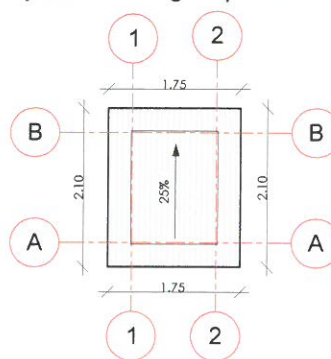
WC public Halta Aghireș - Plan învelitoare
