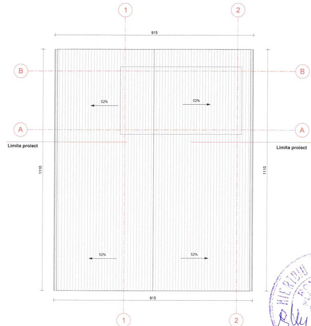
Cabină de pază barieră km 507+978 Baciu - Plan învelitoare
