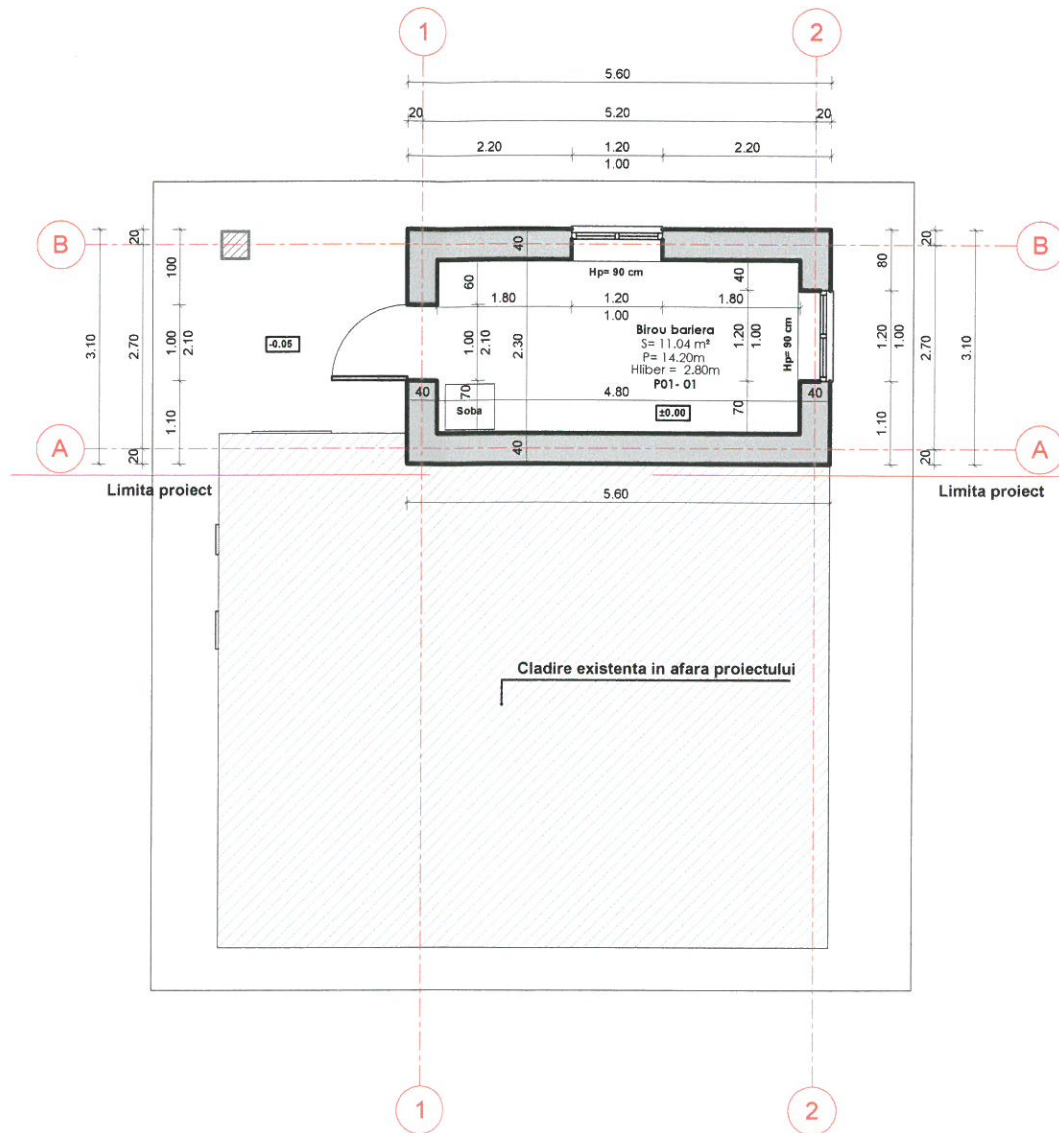
Cabină de pază barieră km 507+978 Baciu - Plan parter
