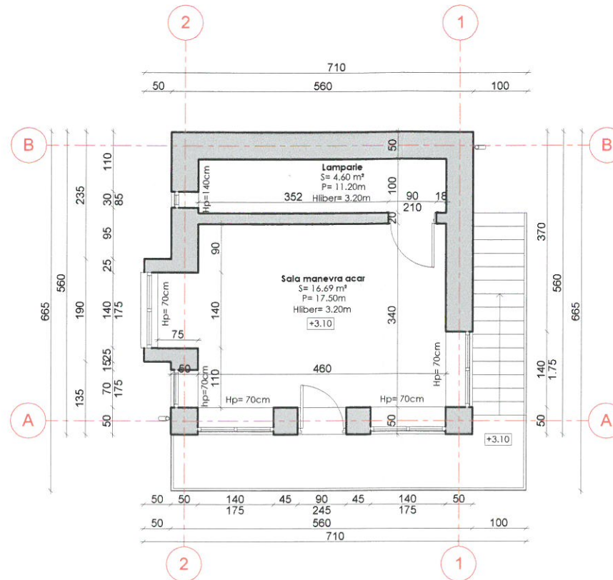
Cabină de centralizare Nr. 1 Ciucea - Plan etaj
