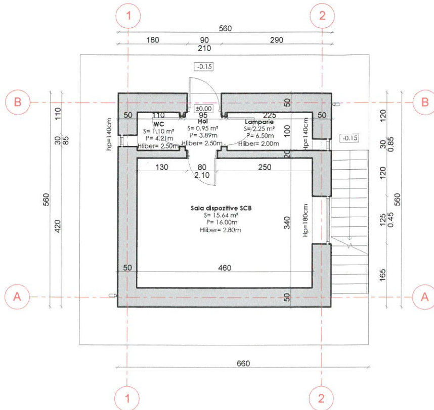
Cabina de centralizare Nr. 1 Ciucea - Plan parter
