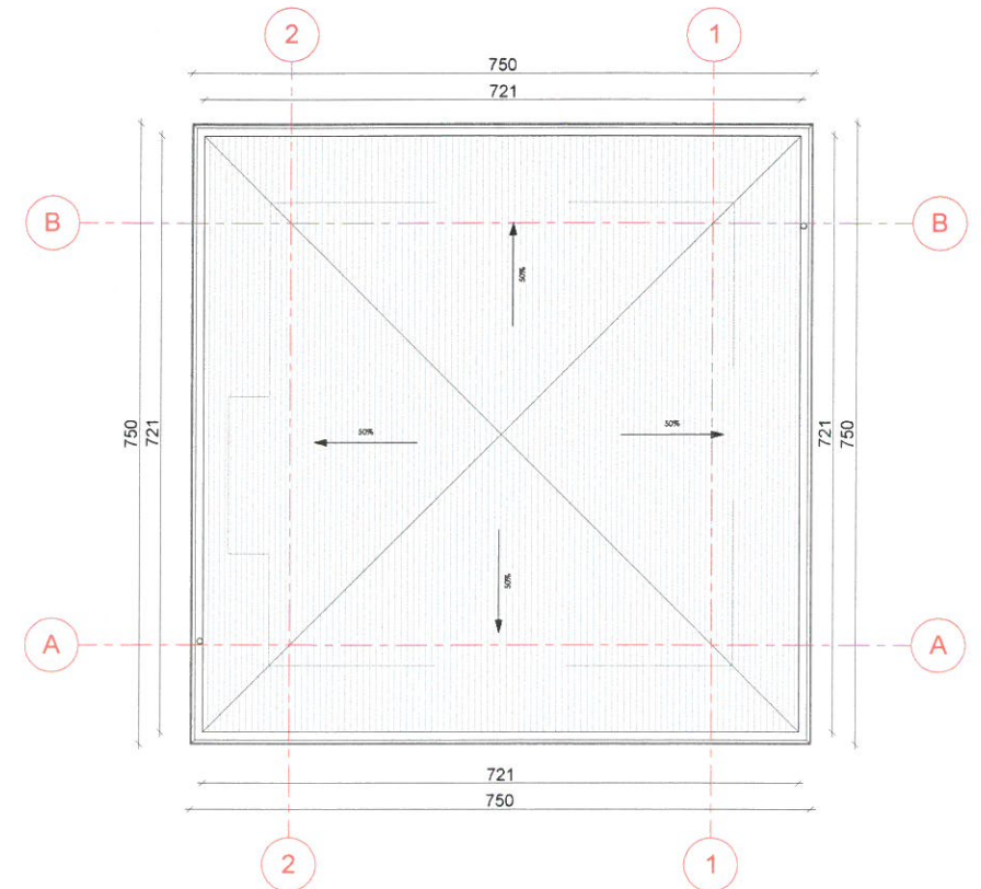
Cabină de centralizare Nr. 1 Ciucea - Plan învelitoare
