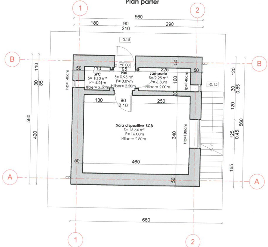
Cabină de centralizare Nr. 2 Clucea - Plan parter
