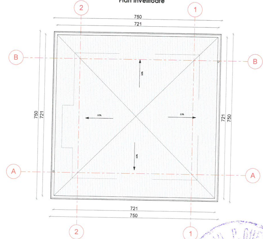
Cabină de centralizare Nr. 2 Clucea - Plan învelitoare
