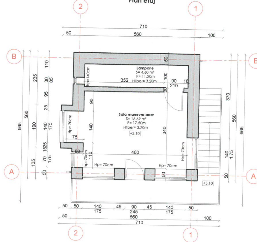
Cabină de centralizare Nr. 2 Clucea - Plan etaj
