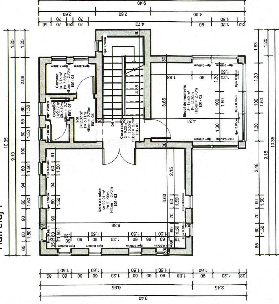
Plan etaj 1
