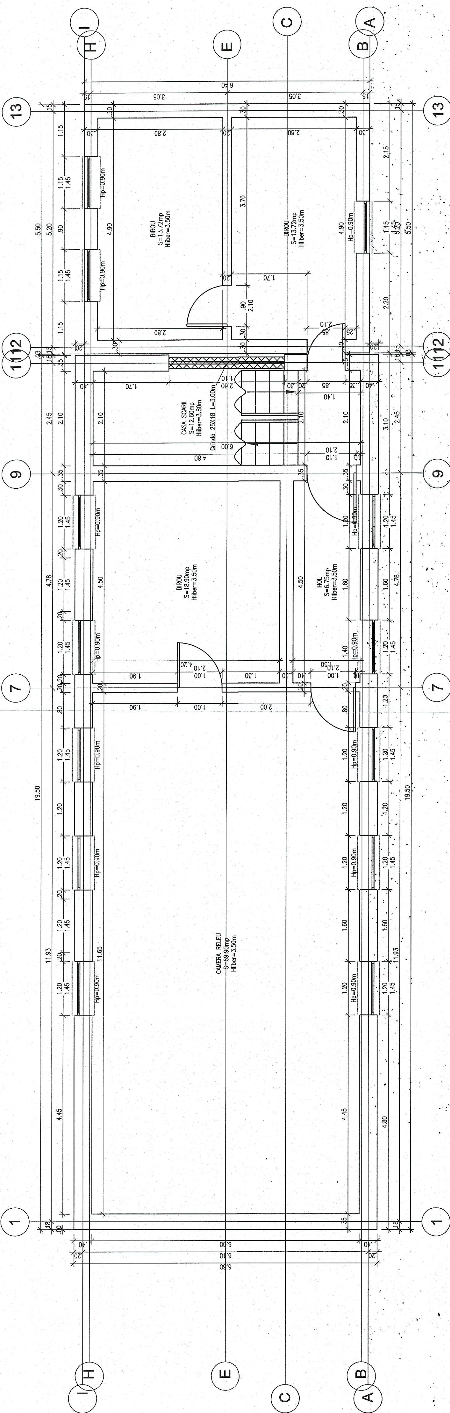
PLAN ETAJ 1 H.util=3.50m
