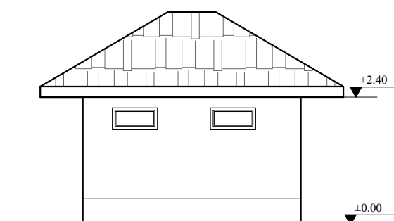
Vedere principala/ Main facade sc 1:100
