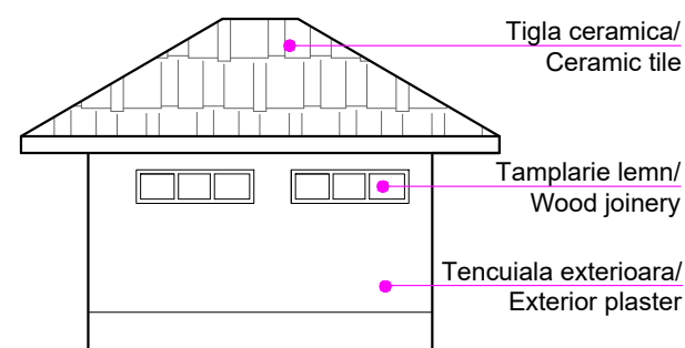
Vedere secundara/ Secondary facade sc 1:100
