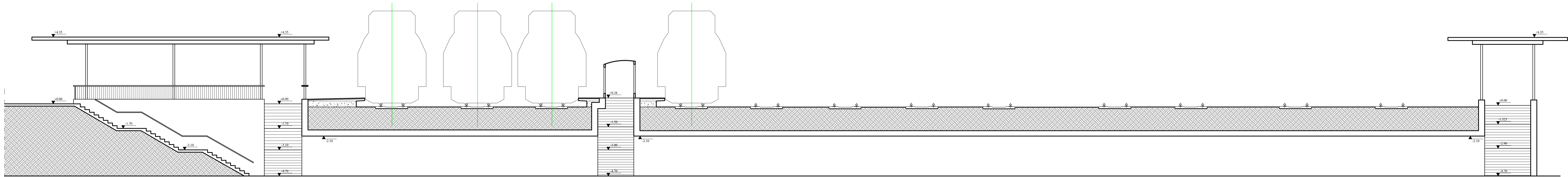
SECTIUNE LONGITUDINALA - RELEVU sc 1:100 Stația București Chitila - Tunel Pietonal - Sectiune Longitudinală - Relevu București Chitila Station - Pedestrian Tunnel - Longitudinal Section - Survey
