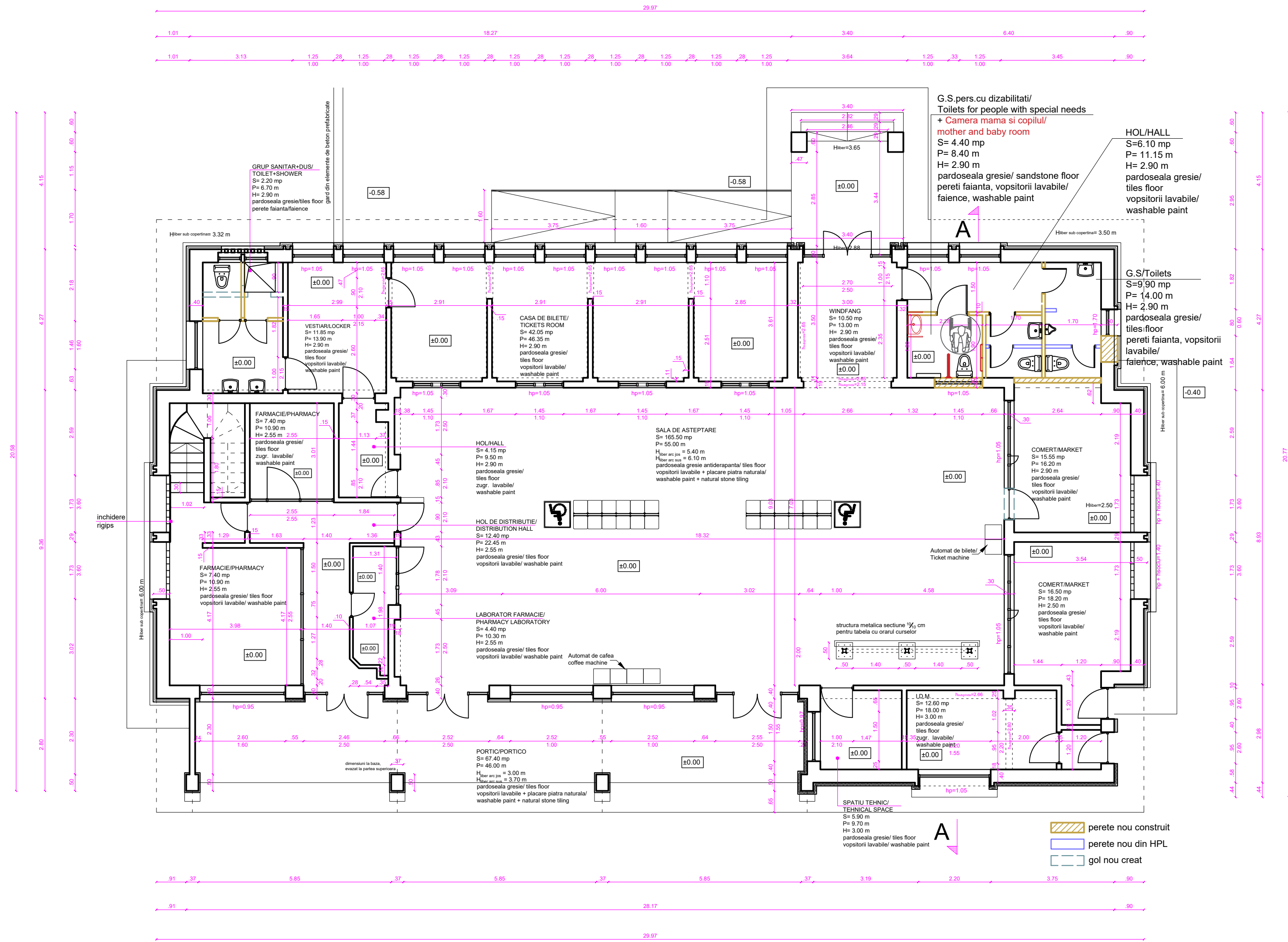
Cladire Calatori BASARAB plan parter
