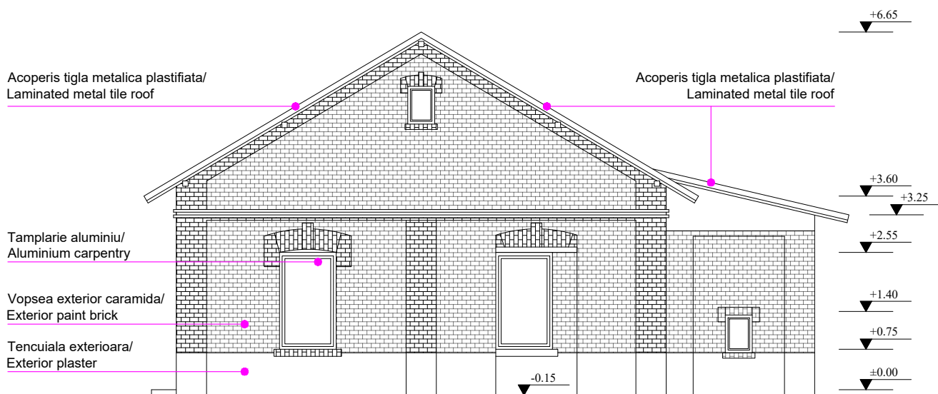
Cladire Politie/Police building Vedere laterală/Side facade sc 1:100
