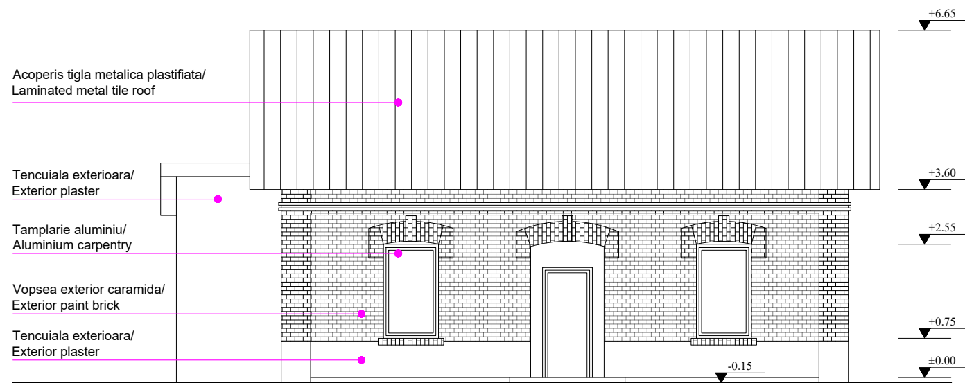
Cladire Politie/Police building Vedere principală/Main facade sc 1:100
