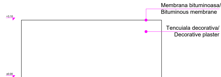
Clădire post mișcare 5/ Post movement building 5 Vedere secundară/Secondary view sc 1:100
