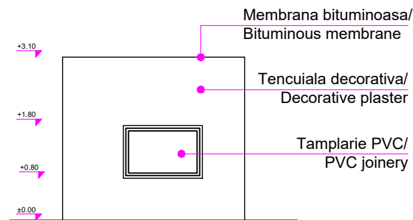
Clădire post mișcare 5/ Post movement building 5 Vedere laterală dreapta/Right side view sc 1:100
