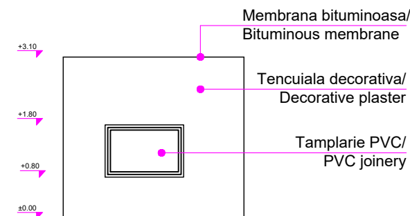
Clădire post mișcare 5/ Post movement building 5 Vedere laterală stânga/Left side view sc 1:100
