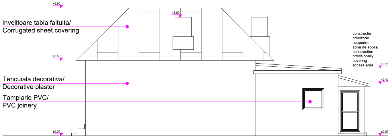
Clădire post mișcare 22/ Post movement building 22 Vedere principală/Main view sc 1:100
