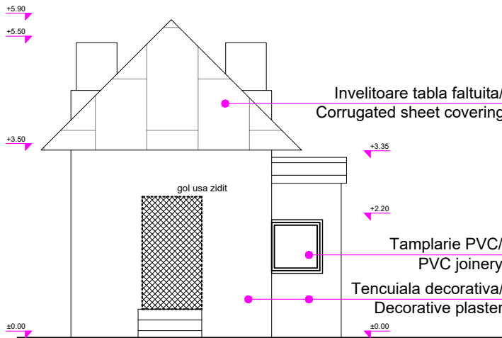
Clădire post mișcare 22/ Post movement building 22 Vedere laterală/Side view sc 1:100
