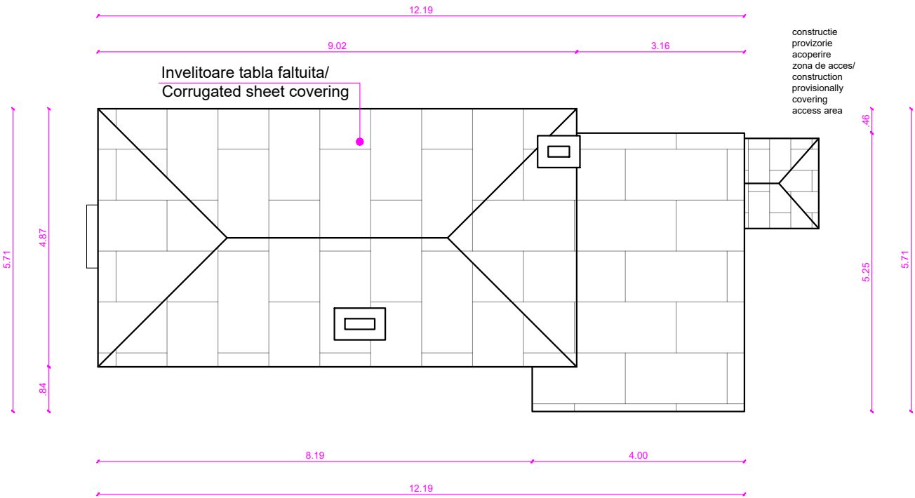
Clădire post mișcare 22/ Post movement building 22 Plan învelitoare/Cover plan sc 1:100 A construita = 25.60 mp A desfasurata = 25.60 mp P = 21.90 m
