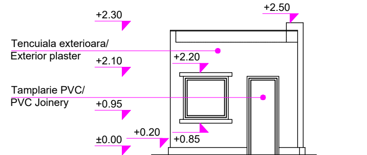
Cabină acari post 5/ Pointsman's Cabin 5 Vedere laterală stânga/ Left Side View sc 1:100
