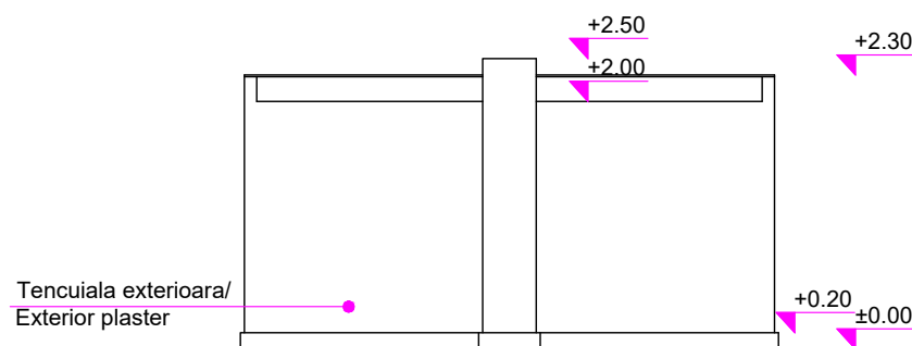
Cabină acari post 5/ Pointsman's Cabin 5 Vedere secundară/ Side View sc 1:100
