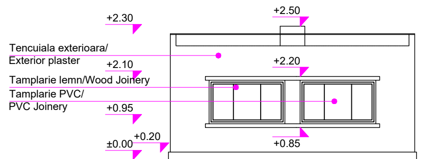
Cabină acari post 5/ Pointsman's Cabin 5 Vedere principală/Main View sc 1:100
