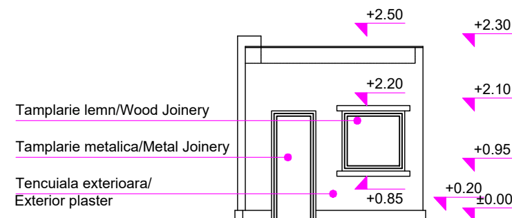
Cabină acari post 5/ Pointsman's Cabin 5 Vedere laterală dreapta/ Right Side View sc 1:100
