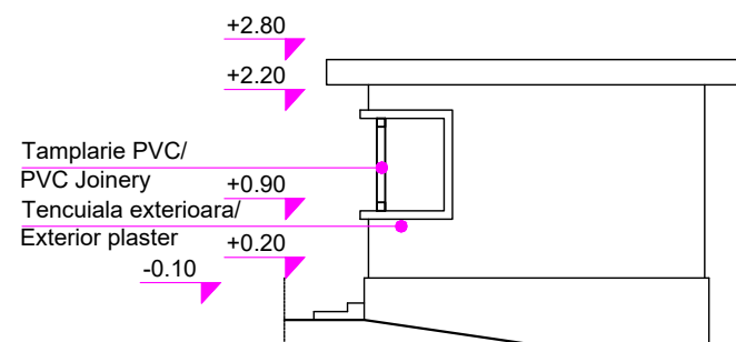
Cabină acari 2/Pointsman's Cabin 2 Vedere laterală dreapta/Right Side View sc 1:100
