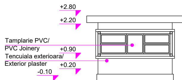
Cabină acari 2/Pointsman's Cabin 2 Vedere principală/ Main View sc 1:100
