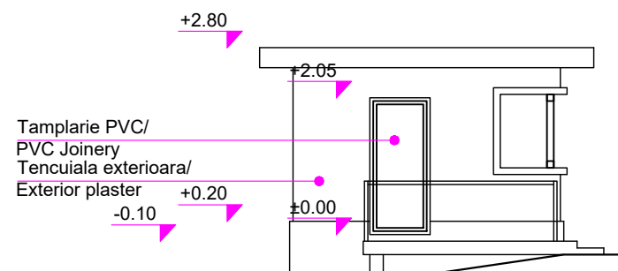
Cabină acari 2/Pointsman's Cabin 2 Vedere laterală stânga/ Left Side View sc 1:100
