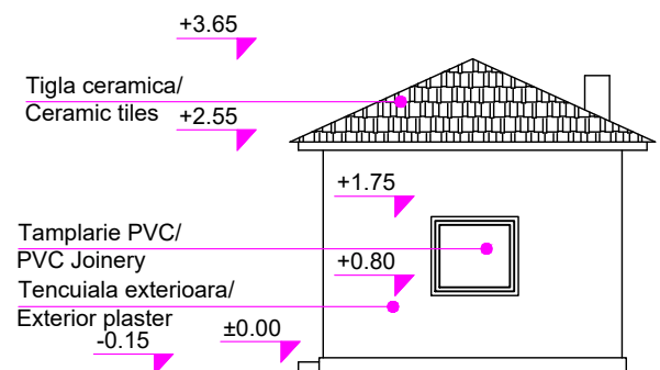
Cabină acari 14/ Pointsman's Cabin 14 Vedere principală/ Main View sc 1:100
