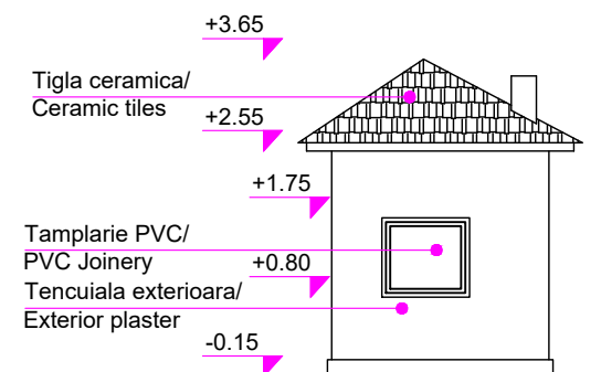
Cabină acari 14/ Pointsman's Cabin 14 Vedere laterală dreapta/ Main View sc 1:100
