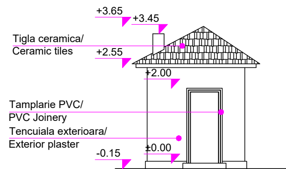
Cabină acari 14/Pointsman's Cabin 14 Vedere laterală stânga/ Left side view sc 1:100
