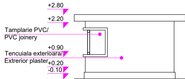
Cabină acari post 4/Pointsman's Cabin 4 Vedere laterală dreapta/ Right side view sc 1:100
