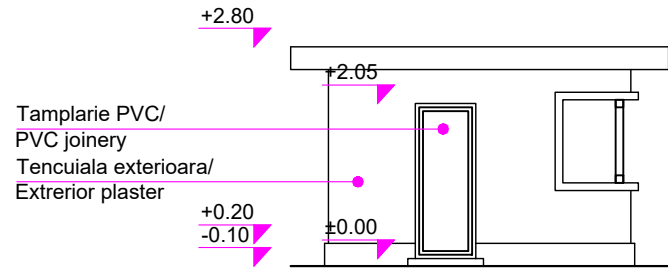
Cabină acari post 4/Pointsman's Cabin 4 Vedere laterală stânga/ Left side view sc 1:100
