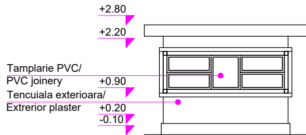
Cabină acari post 4/Pointsman's Cabin 4 Vedere principală/ Main View sc 1:100
