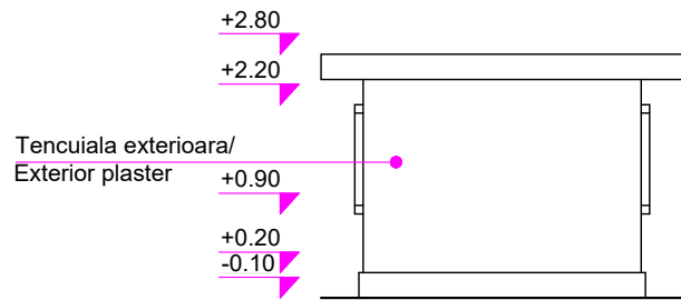
Cabină acari post 16/ Pointsman's Cabin 16 Vedere secundară/ Secondary View sc 1:100
