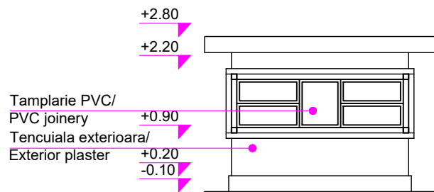
Cabină acari post 16/Pointsman's Cabin 16 Vedere principală/ Main view sc 1:100
