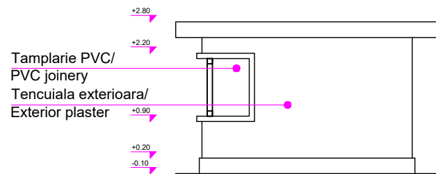
Cabină acari post 16/Pointsman's Cabin 16 Vedere laterală dreapta/ Right side view sc 1:100
