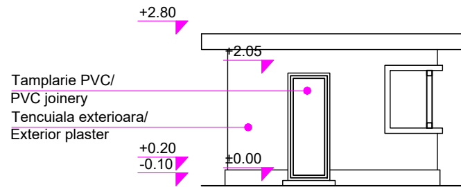
Cabină acari post 16/ Pointsman's Cabin 16 Vedere laterală stânga/ Left side view sc 1:100
