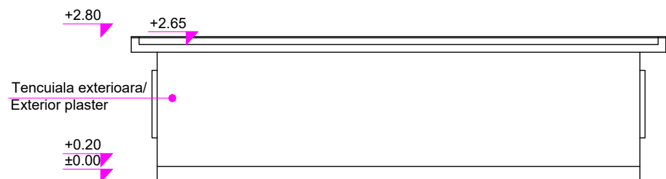
Cabină acari post 6/ Pointsman's Cabin 6 Vedere secundară/ Secondary view sc 1:100
