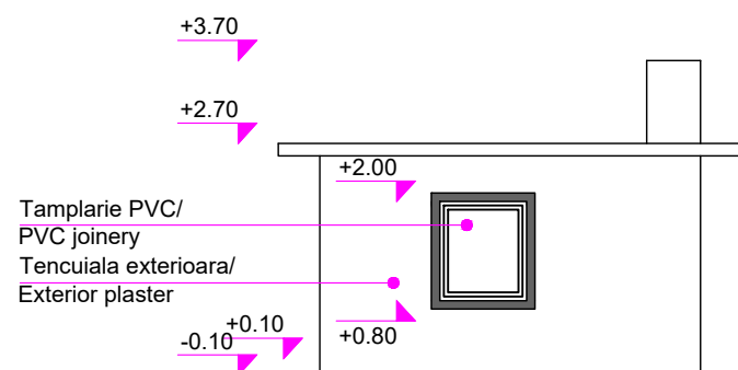
Cabină acari post 10/Pointsman's Cabin 10 Vedere principală/Main View sc 1:100
