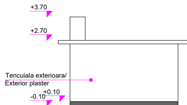
Cabină acari post 10/Pointsman's Cabin 10 Vedere secundară/ Side view sc 1:100
