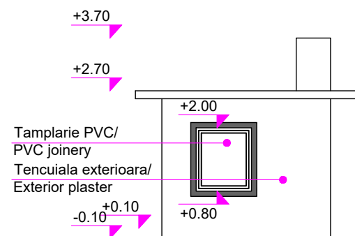
Cabină acari post 10/Pointsman's Cabin 10 Vedere laterală dreapta/Right side view sc 1:100
