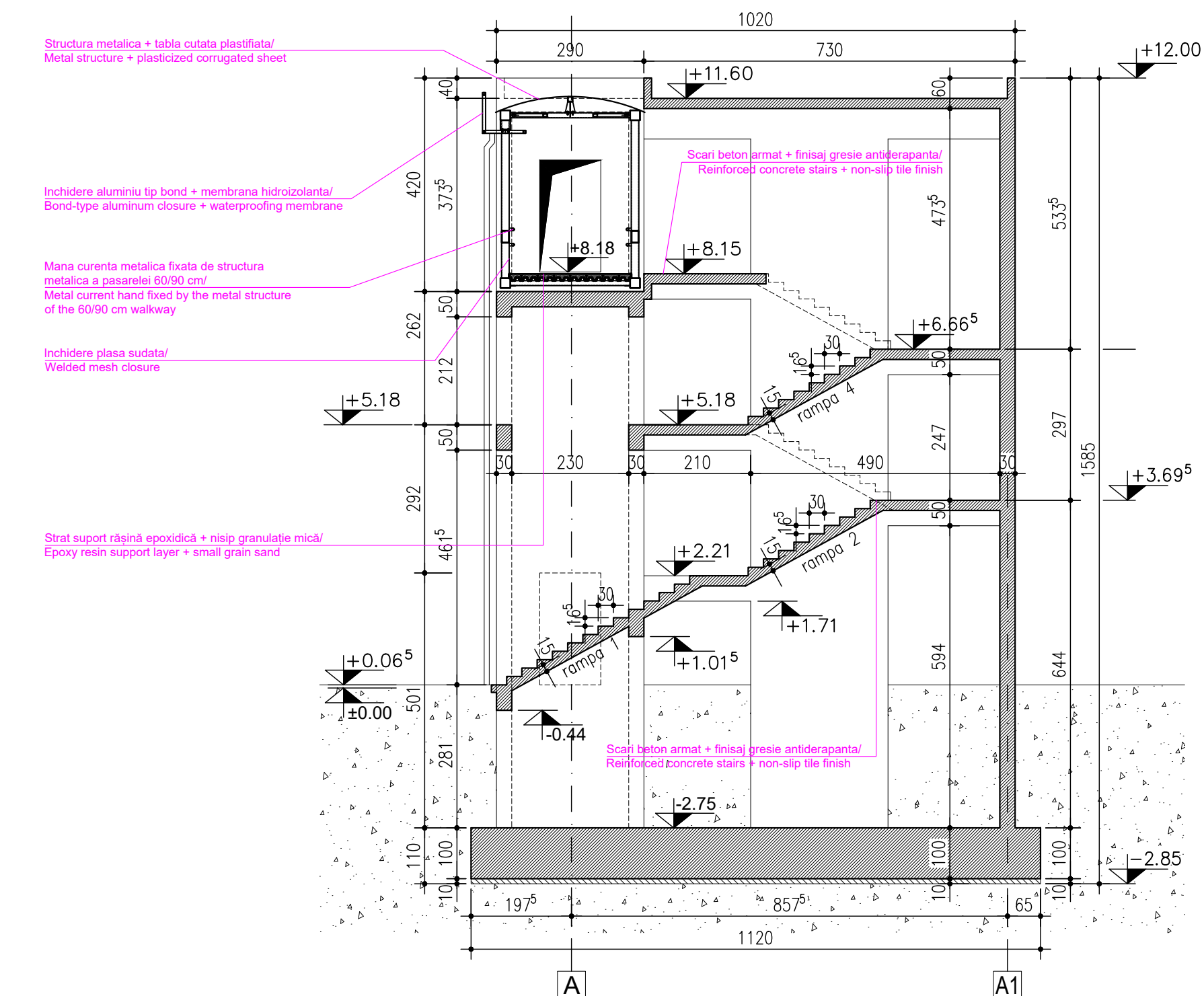
Sețiune transversala / Cross section Scara/Scale 1:100
