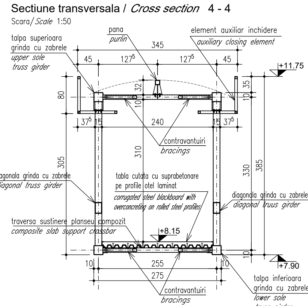
Sección transversal / Cross section 4 - 4
