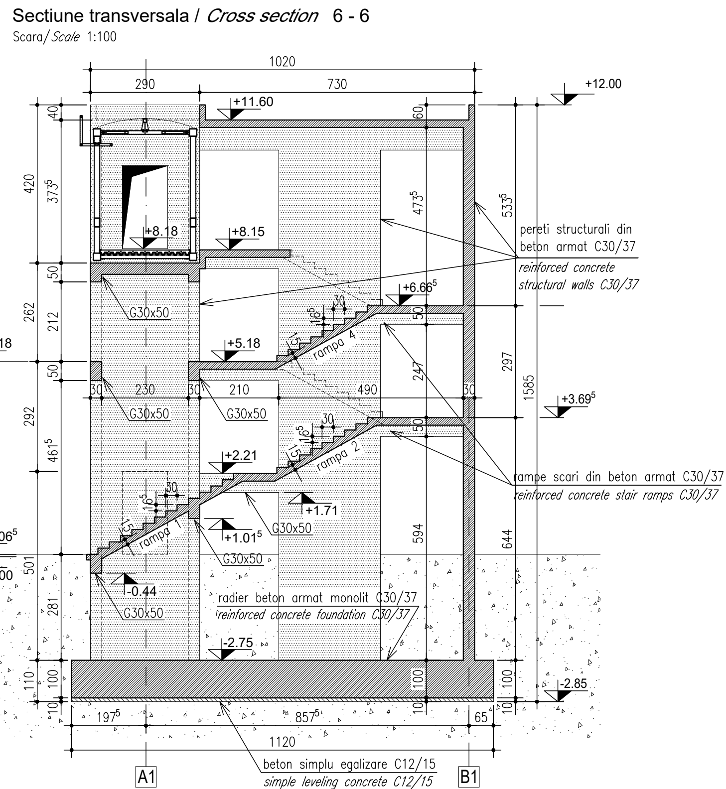
Sección transversal / Cross section 6 - 6
