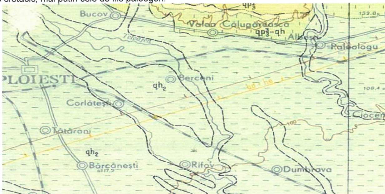
Fragment din harta geologica Ploiesti
