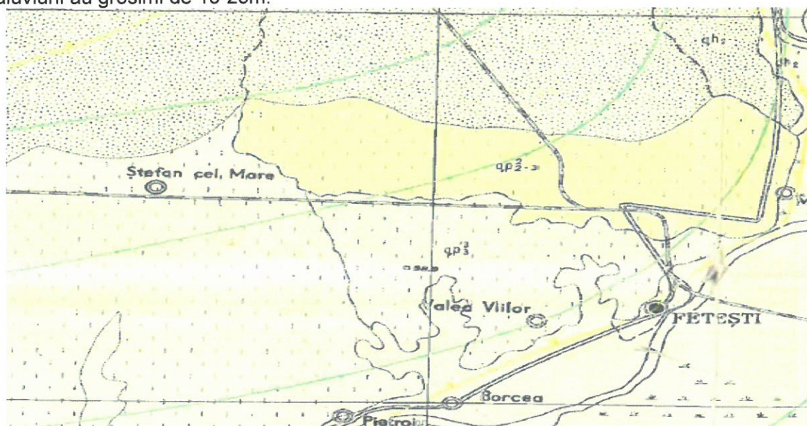
Fragmente din harta geologica Calarasi. Zona Baraganu
