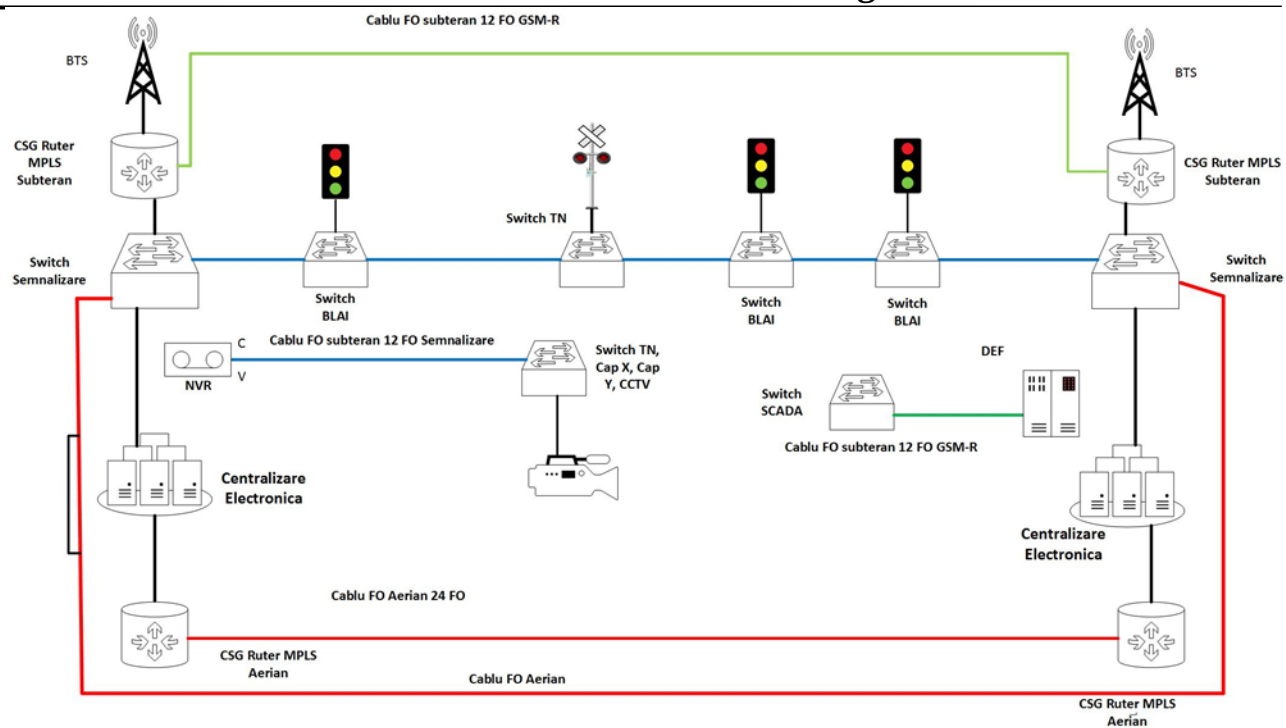
Schema de principiu pentru conectarea BLAI pe FO
