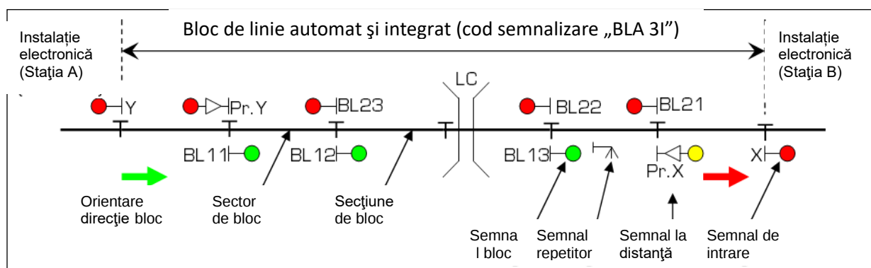
Fig. 3 Componente BLAI
