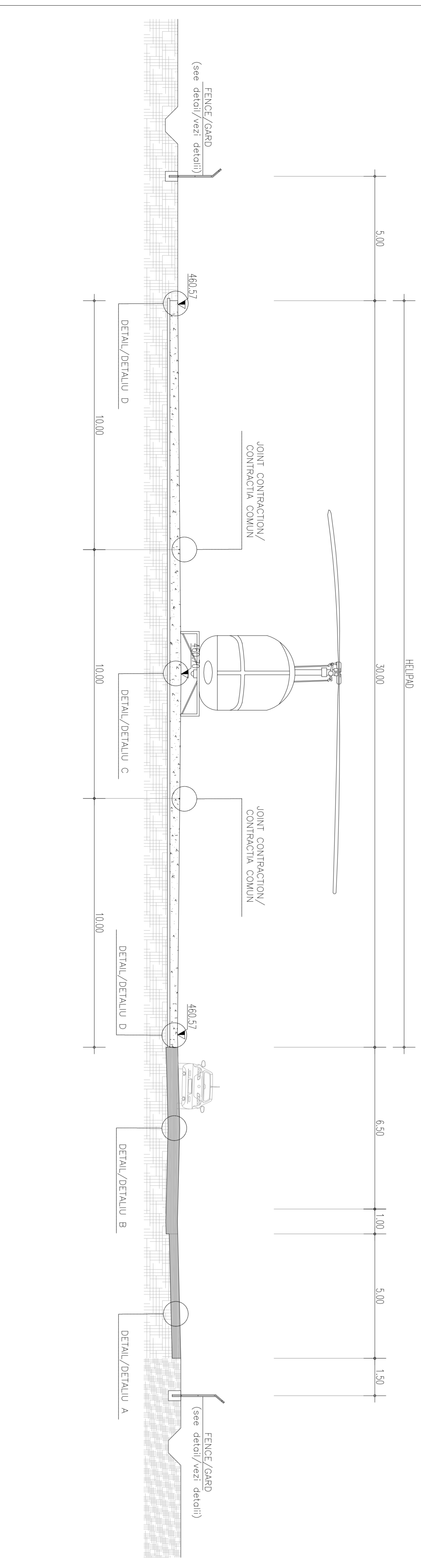
SECTION/SECȚIUNEA A-A Scale/Scara 1:100
