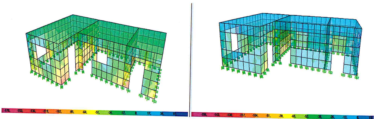
Eforturi secționale \sigma_{22} din seism pe X și Y
