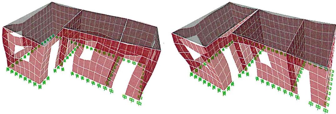
Mod 1 de vibrație ( T_1 = 0.0552 s – translație pe X) și mod 2 ( T_2 = 0.0489 s – translație pe Y)
