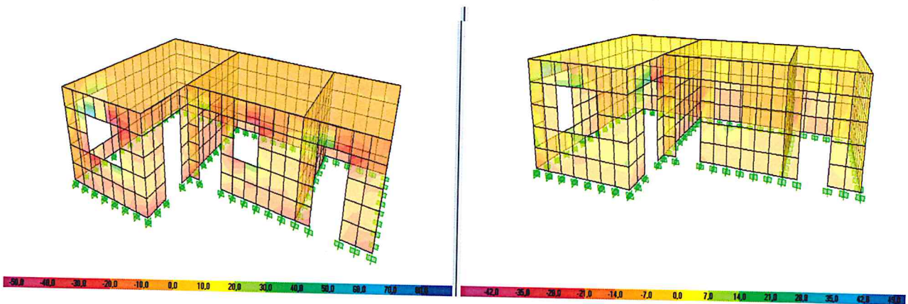
Eforturi secționale \sigma_{11} din seism pe X și Y
