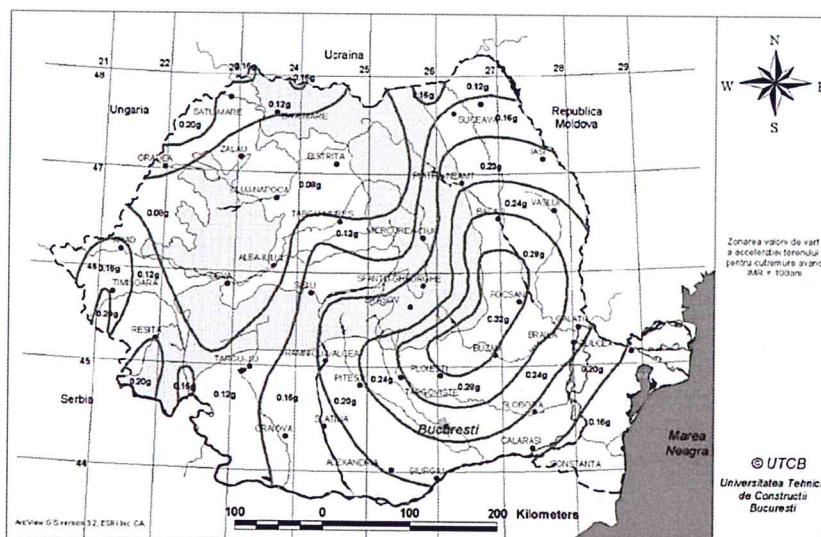
Zonarea teritoriului României în termeni de valori de vârf ale acceleraţiei terenului pentru proiectare a_g pentru cutremure având intervalul mediu de recurenţă \Delta R = 100 ani
