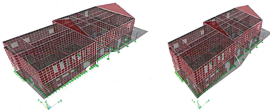
Vedere spațială (3D) clădire
