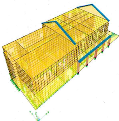
Eforturi secționale \sigma_{22} din seism pe X și Y
