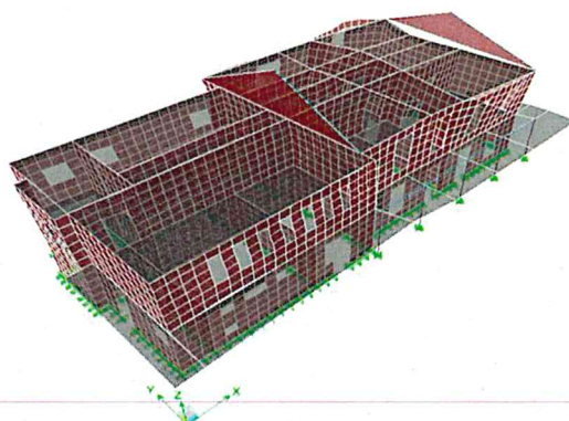
Mod 3 de vibrație ( T_1 = 0.0848 s – torsiune)
