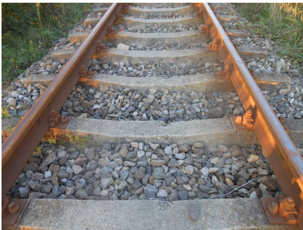
Foto 120 (km 7+200 – km 7+500)
