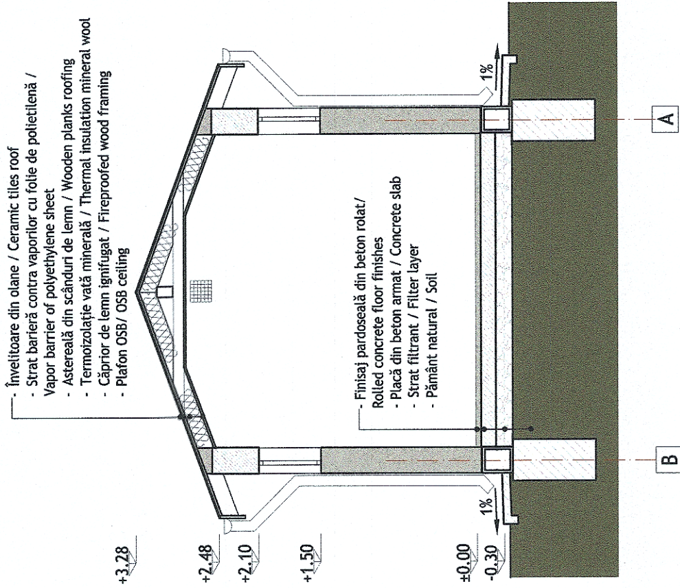
Secțiune transversală 1-1/ Transversal section 1-1
