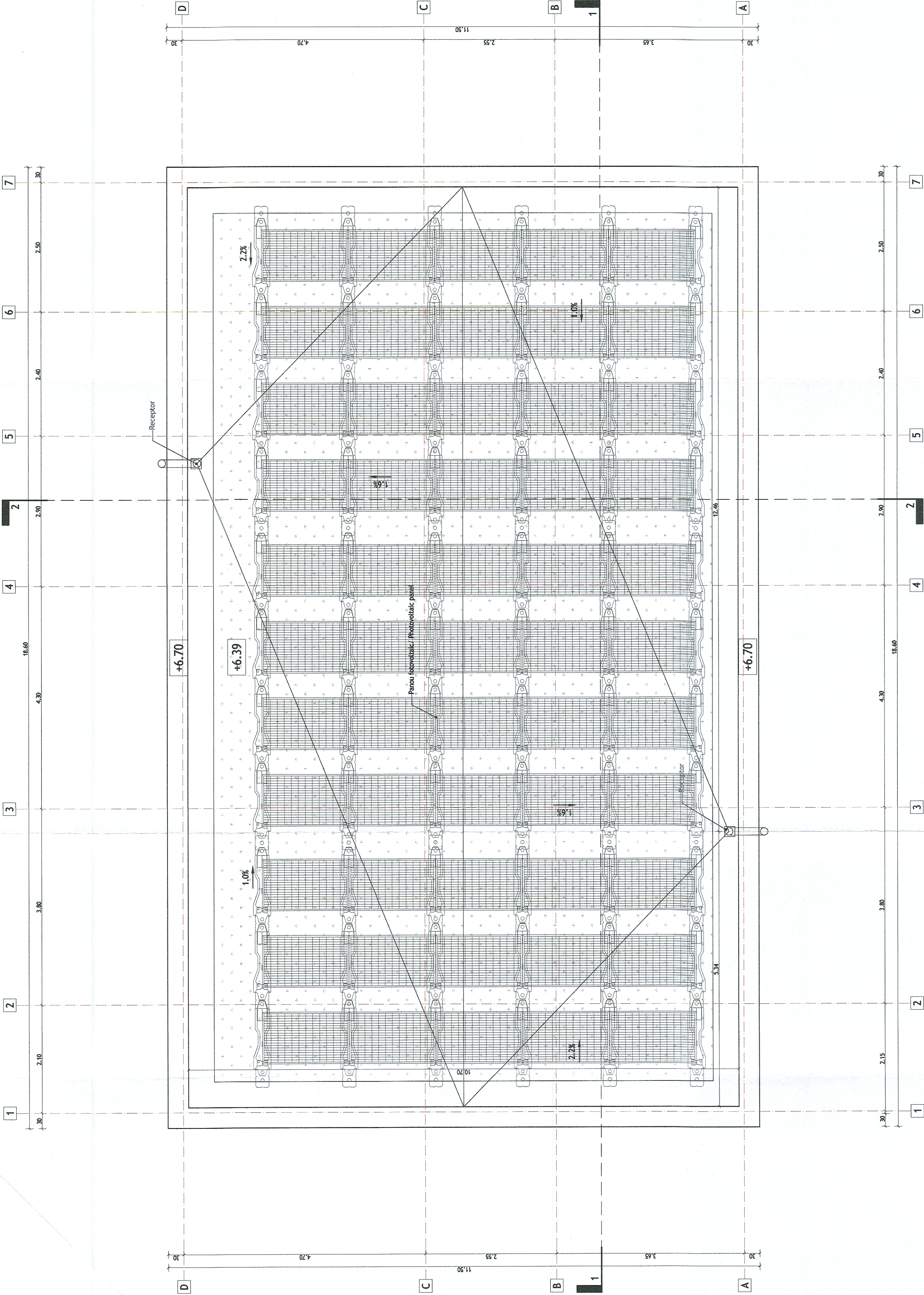
Plan învelitoare / Roof plan
