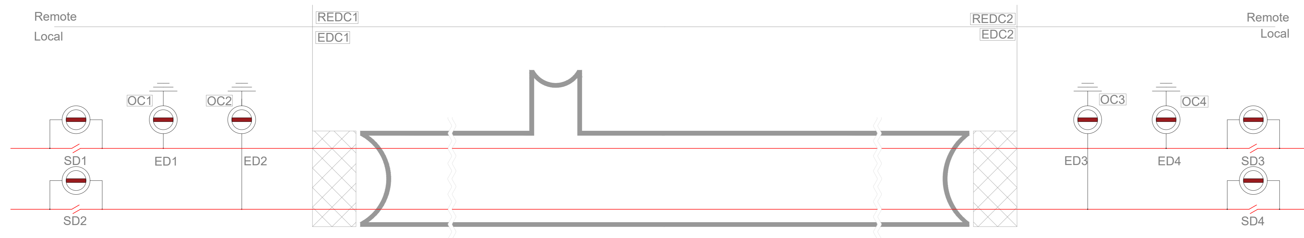
c) Tunnel POARTA I. OCL is energized / Tunelul POARTA I. LC este alimentat
