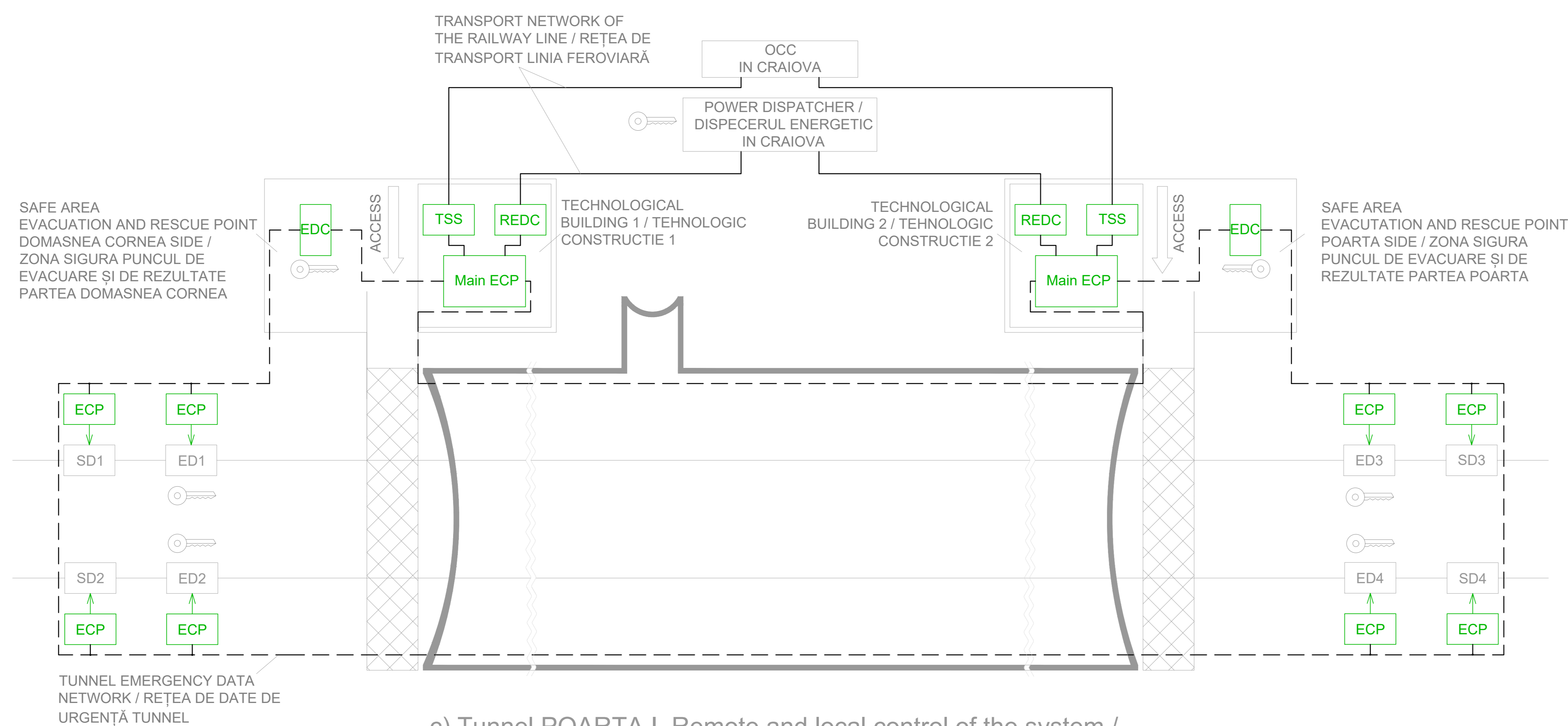
c) Tunnel POARTA I. Remote and local control of the system / Tunelul POARTA I. Controlul de la distanță și local al sistemului
