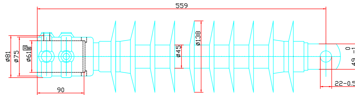
IZOLATOR COMPOZIT PENTRU CONSOLA COMPOSITE INSULATOR FOR CANTILEVER
