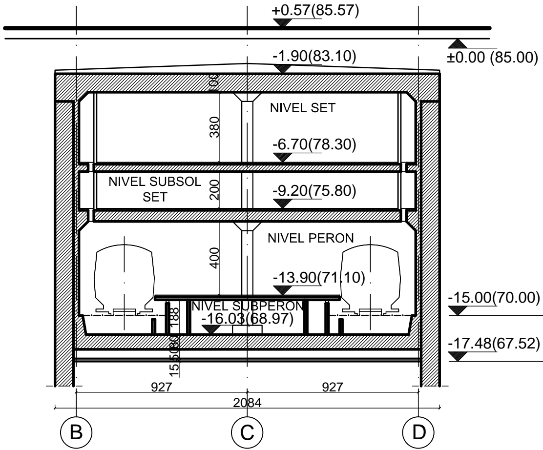
SECȚIUNE TRANSVERSALĂ B-B
