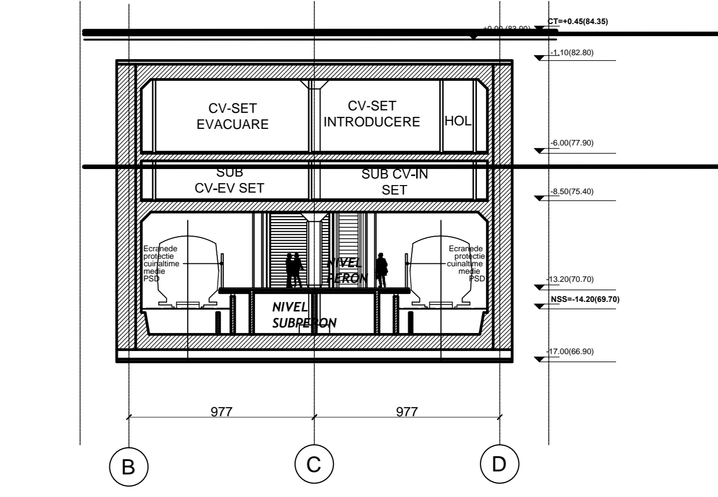
SECTIUNE TRANSVERSALA B-B
