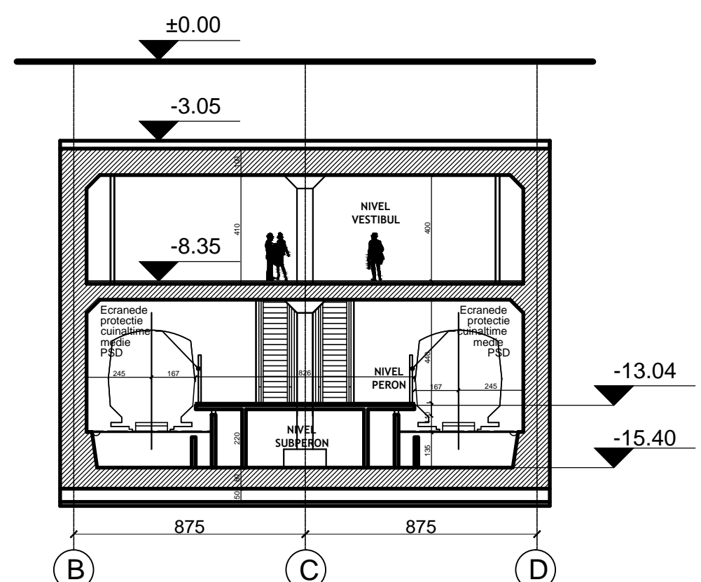
SECȚIUNE TRANSVERSALĂ B-B
