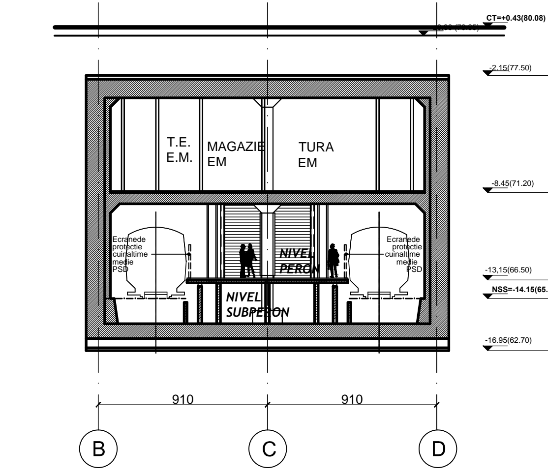
SECȚIUNE TRANSVERSALĂ B-B
