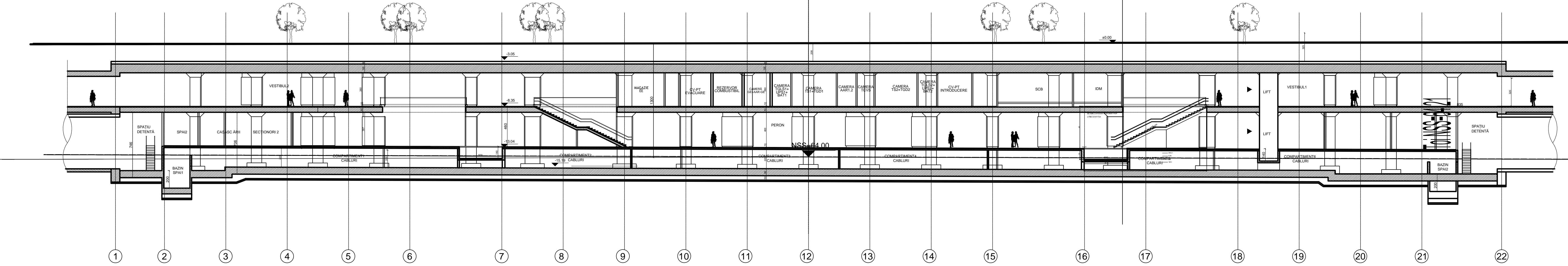
SECȚIUNE LONGITUDINALĂ A-A
