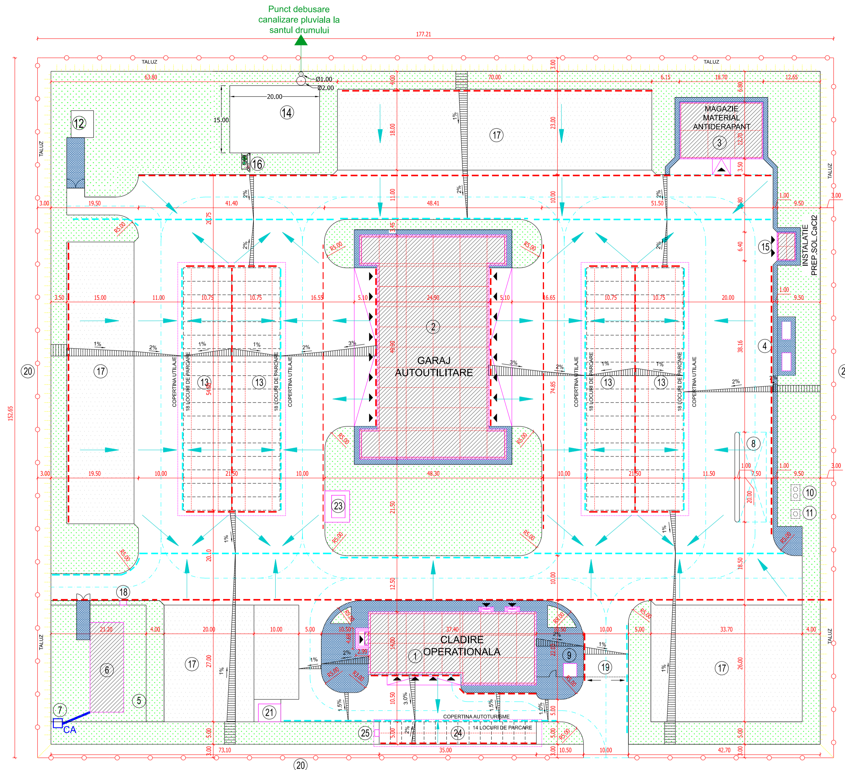
PLAN DE SITUATIE CIC SUPRAFATA DE SPATII VERZI = 7612 MP
