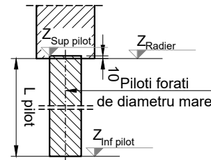
Schita cote de nivel
