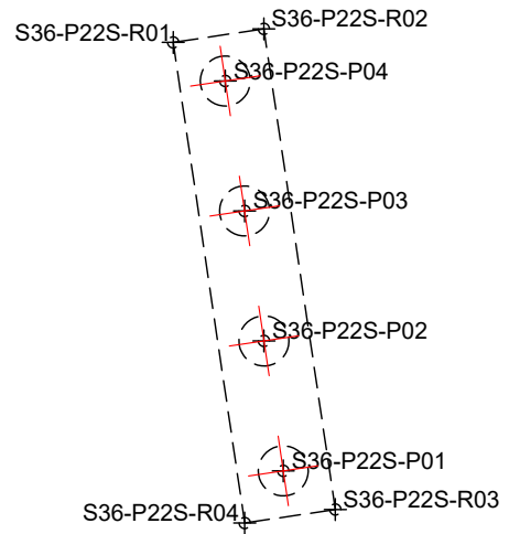
TRASARE RADIER PILA "P22"- fir stanga
