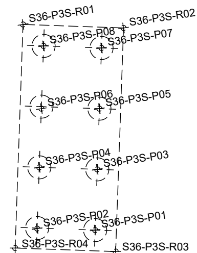
TRASARE RADIER PILA "P3"- fir stanga
