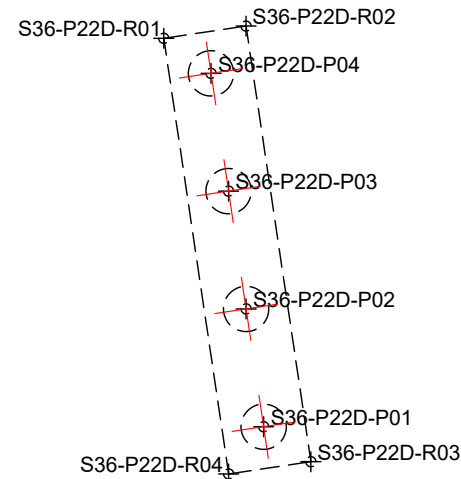
TRASARE RADIER PILA "P22"- fir dreapta
