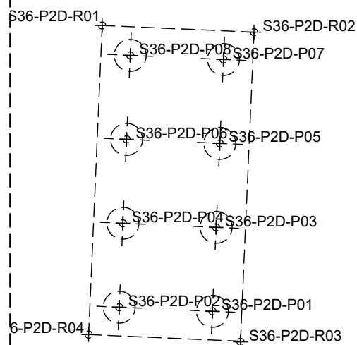
TRASARE RADIER PILA "P2"- fir dreapta
