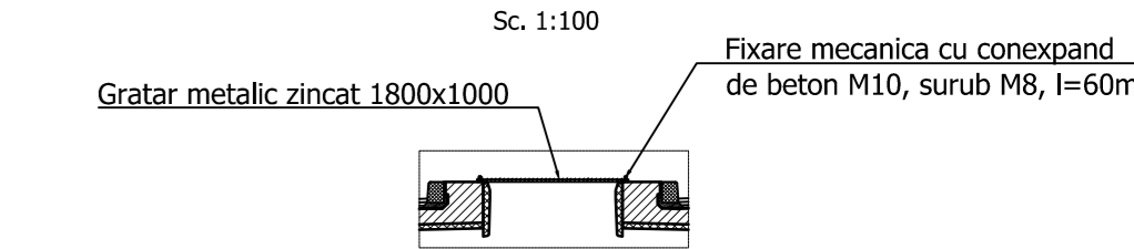
DETALIU FIXARE GRATARE DE PROTECTIE Sc. 1:100
