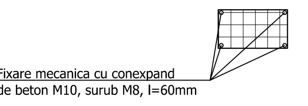
DETALIU FIXARE GRATARE DE PROTECTIE Sc. 1:100
