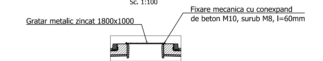
DETALIU FIXARE GRATARE DE PROTECTIE Sc. 1:100
